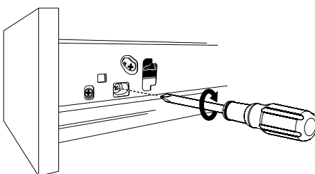
Réglage de la hauteur Height adjustment
