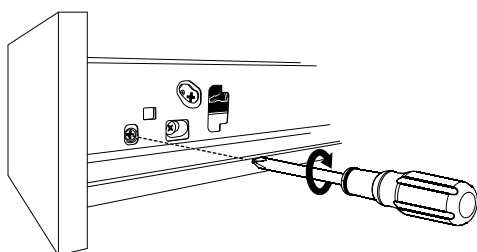
Réglage latéral Side adjustment
