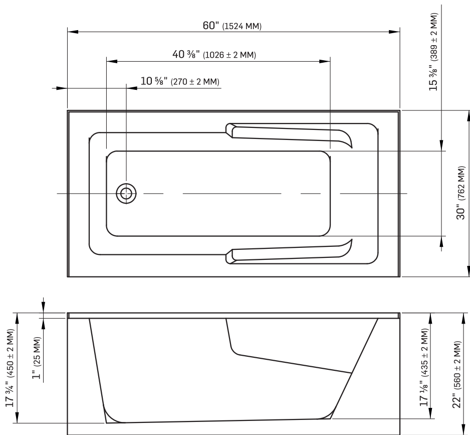
Gabarit 3011217 / 3011218*
