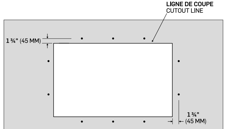
EMPLACEMENT DES TROUS D'ATTACHES SOUS LE COMPTOIR (VUE DU DESSOUS) UNDERMOUNT CLIP HOLE LOCATIONS (UNDERSIDE OF COUNTERTOP)
