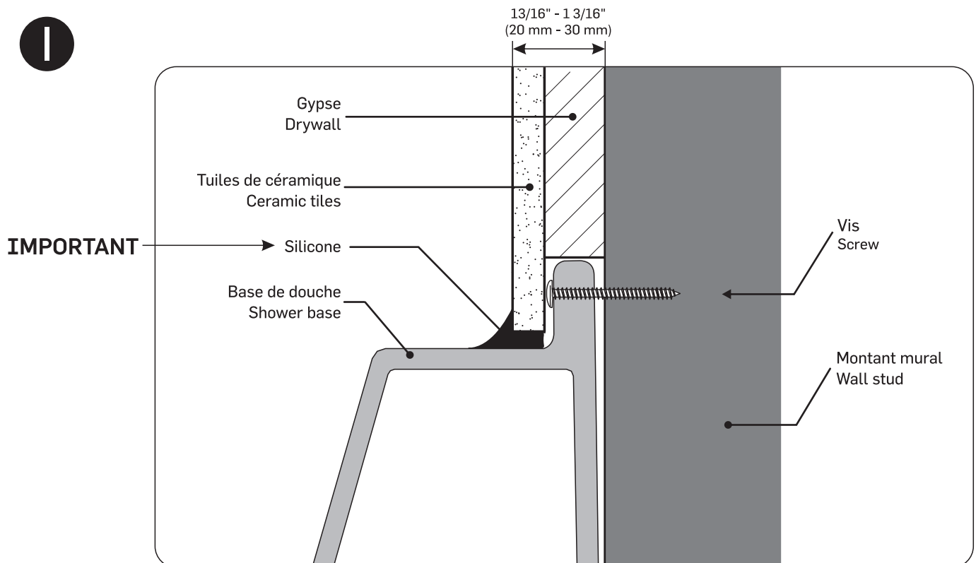
VUE SECTIONNELLE / SIDE SECTION VIEW
